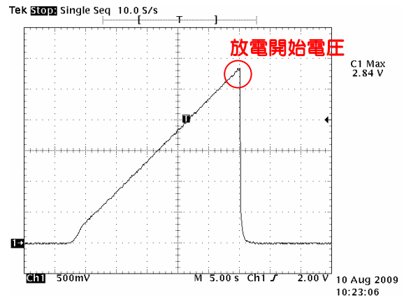
図2 アレスタの動作試験
