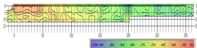
図 2 2.4GHz 信号強度分布
