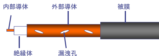
図 1 LCX の構造
